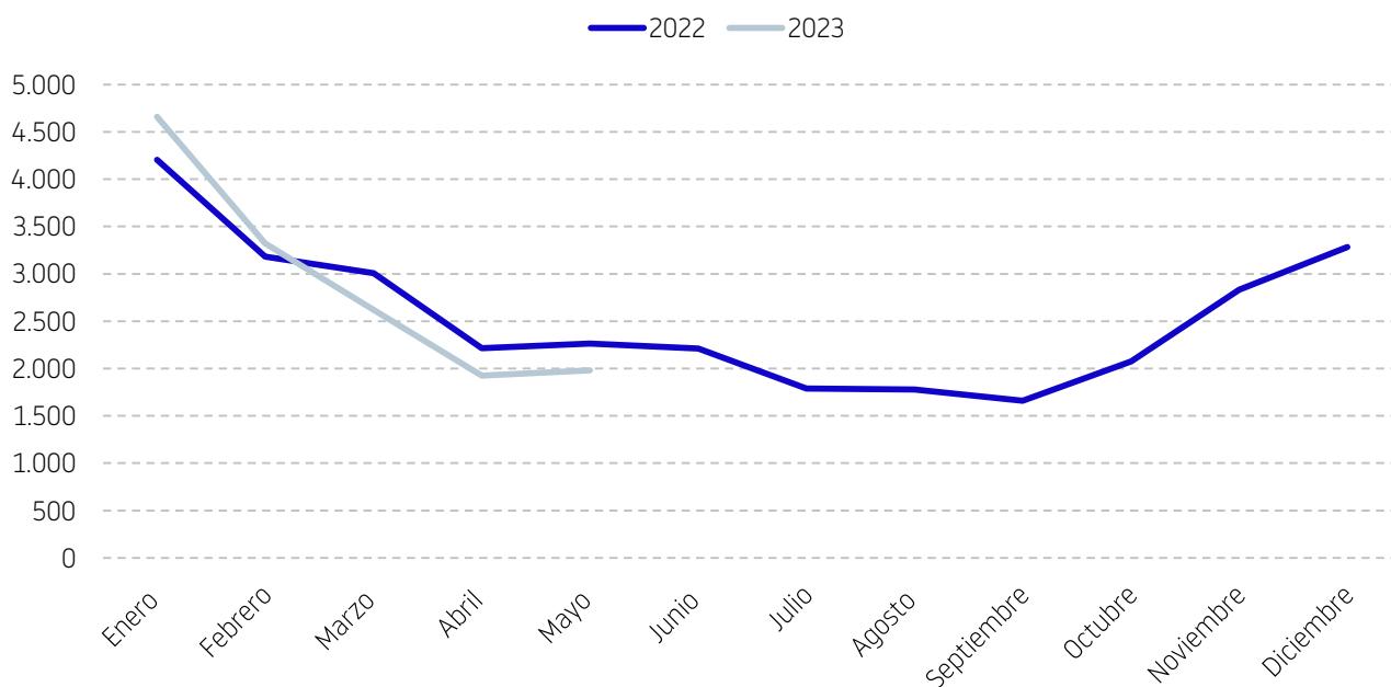
EVOLUCIÓN DISOLUCIONES
